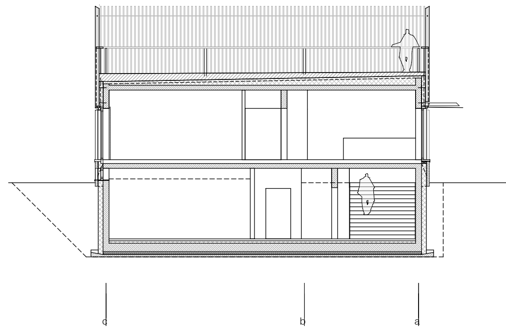
Schnitt D-D
