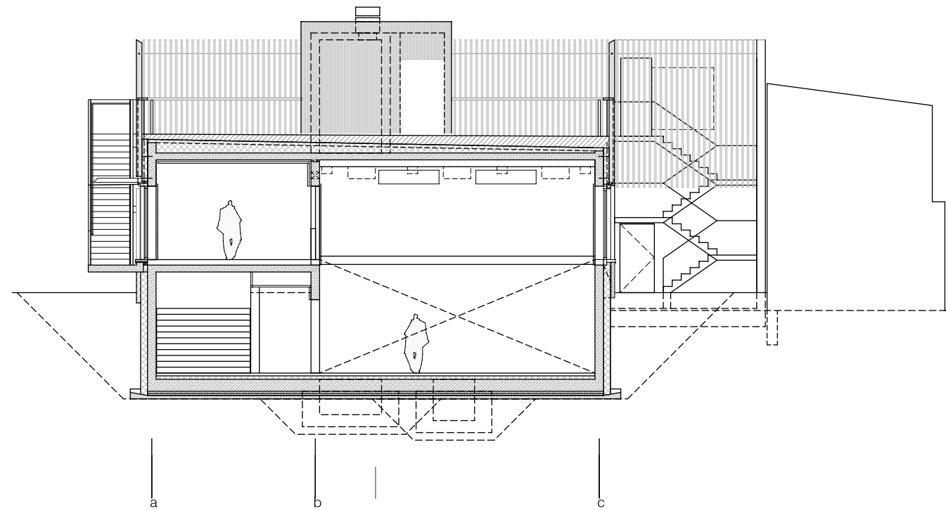
Schnitt C-C
